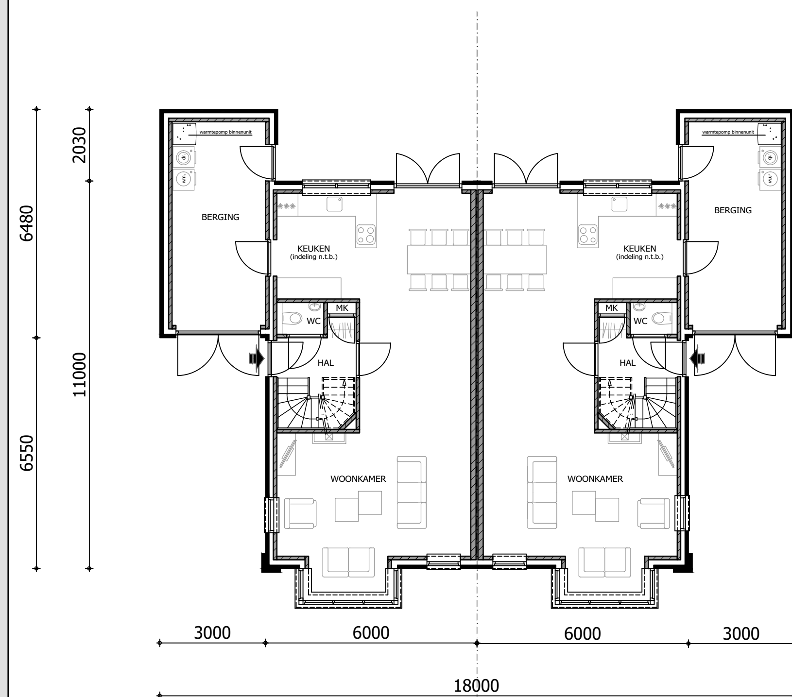
BEGANE GROND
