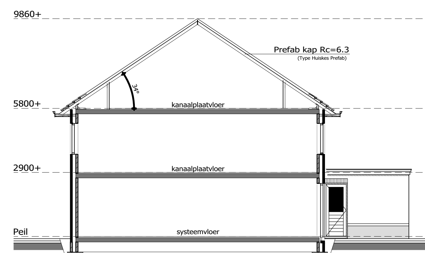
DOORSNEDE
