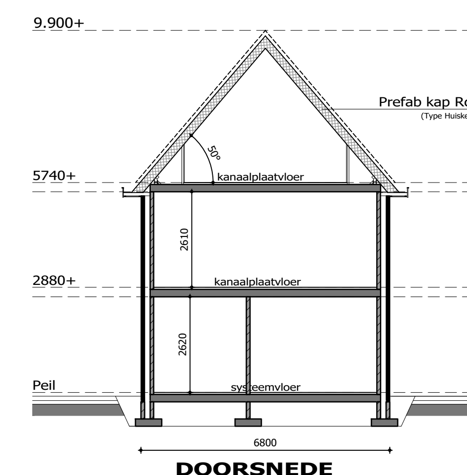
DOORSNEDE
