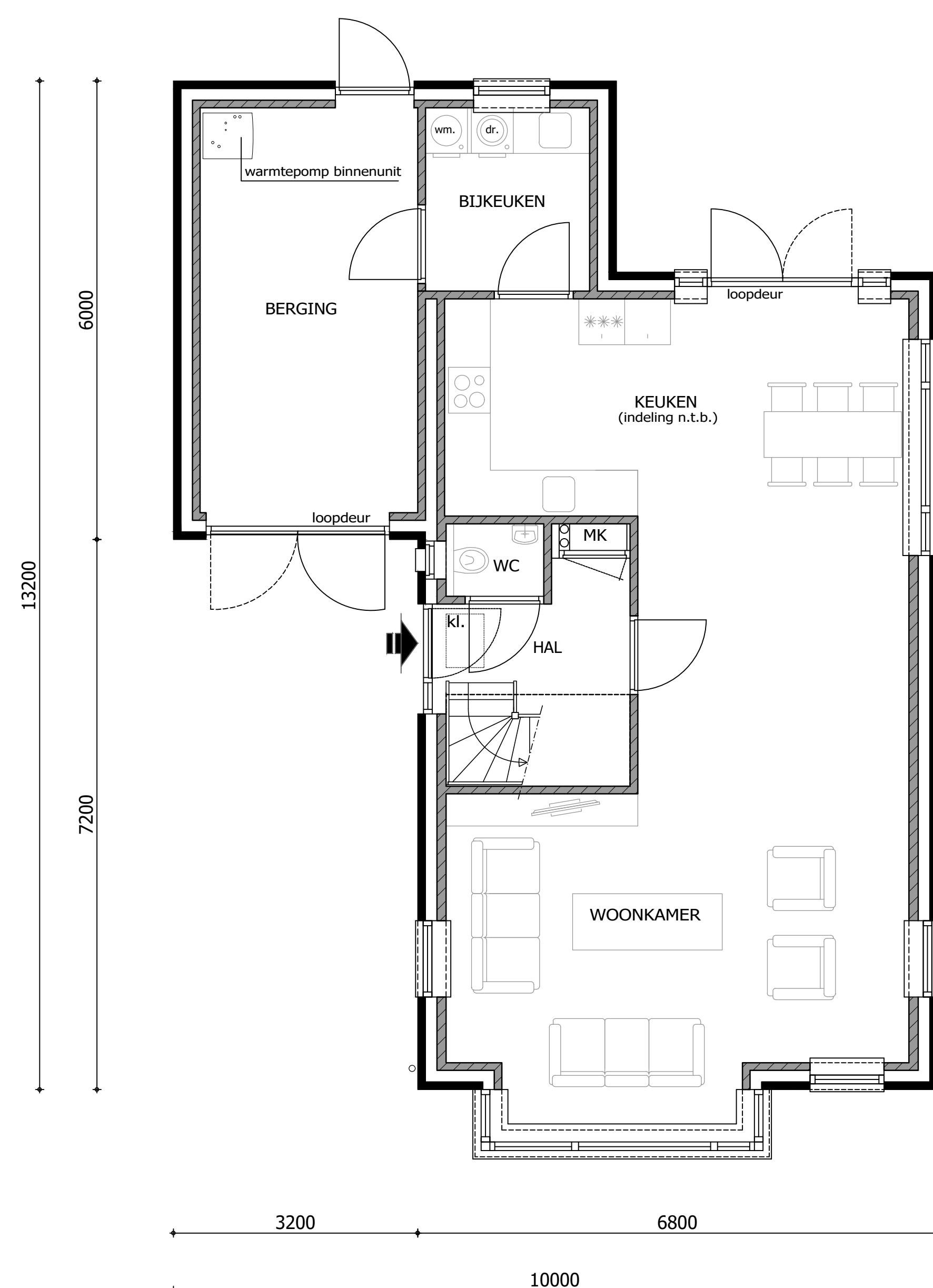
BEGANE GROND
