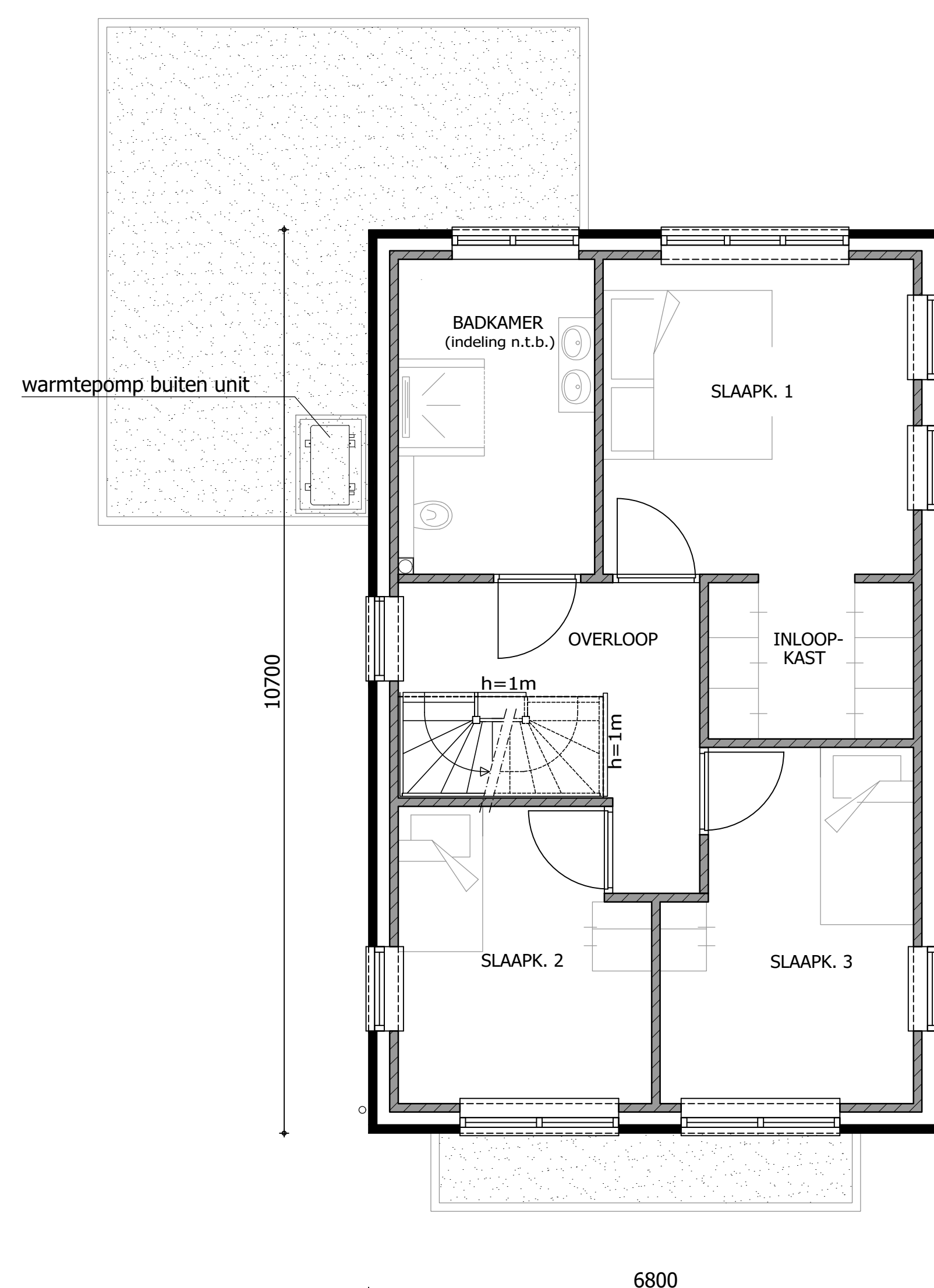
VERDIEPING
