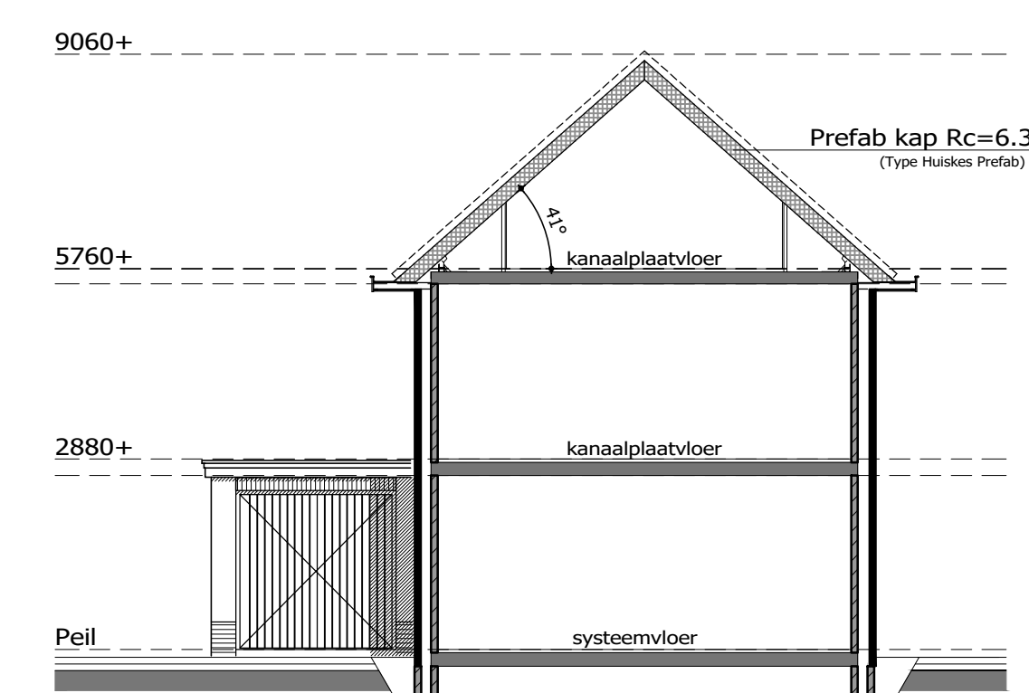
DOORSNEDE A-A
