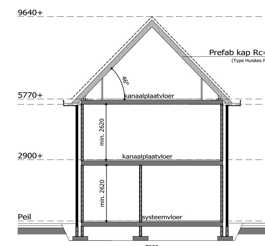
DOORSNEDE
