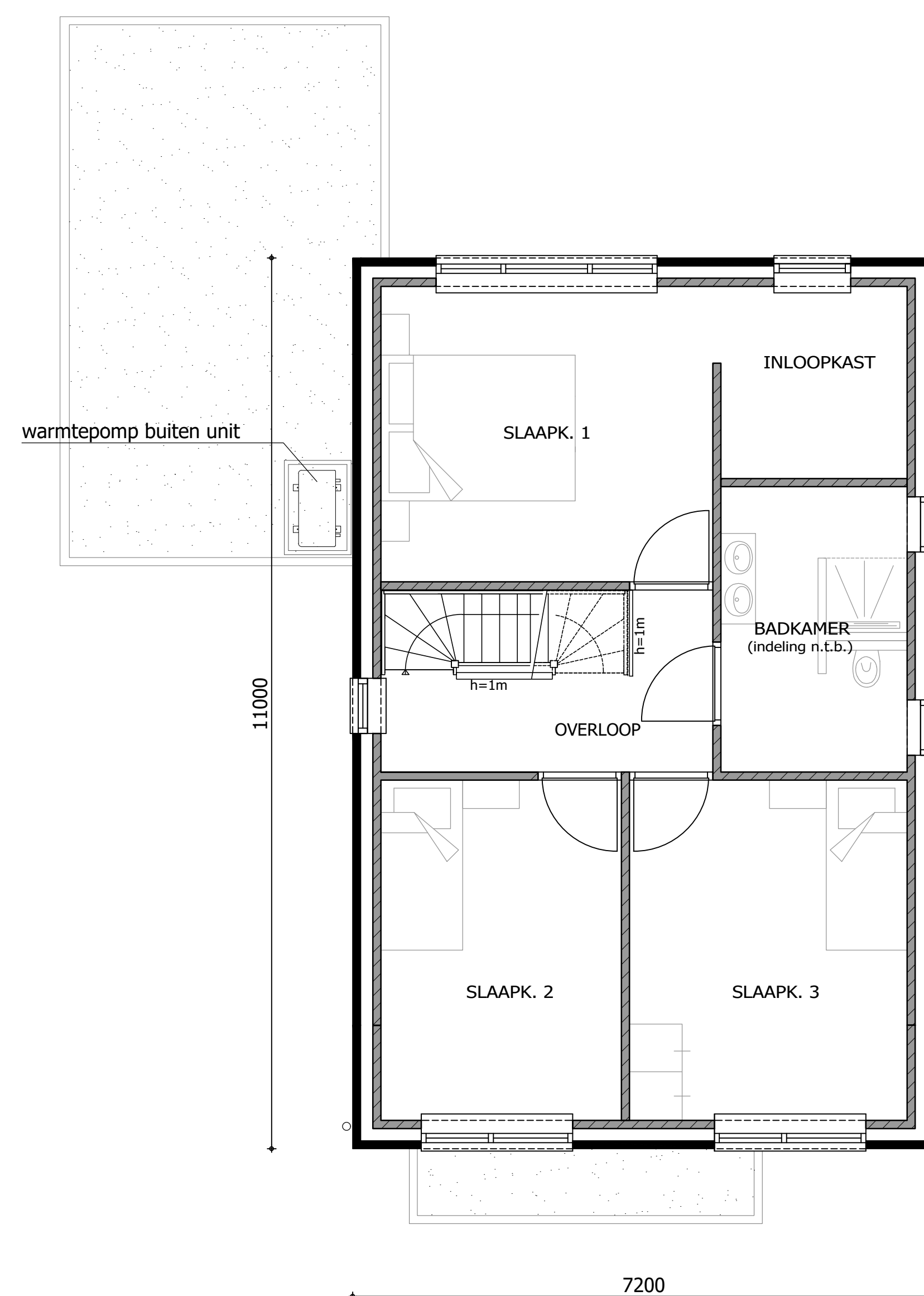
VERDIEPING
