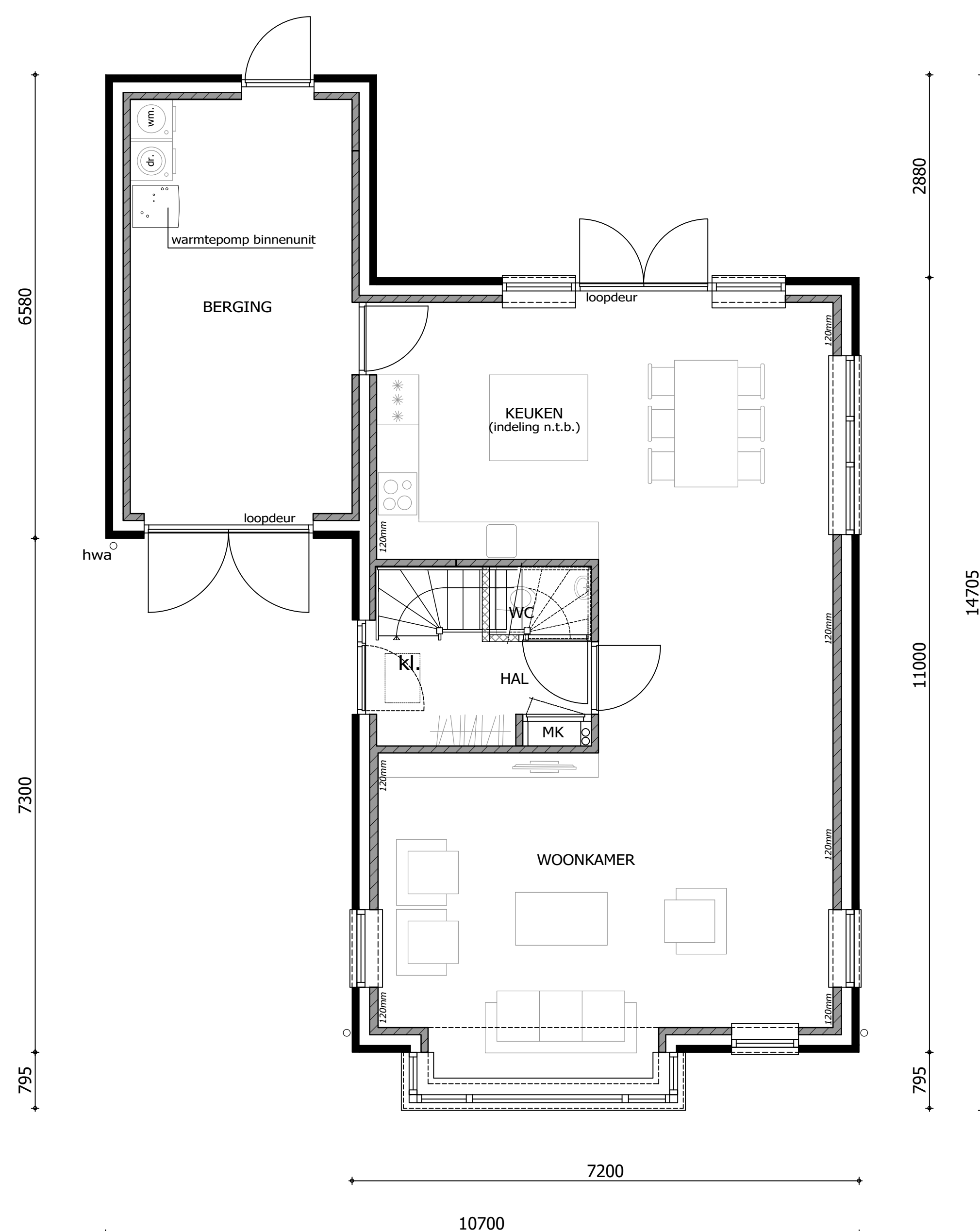
BEGANE GROND
