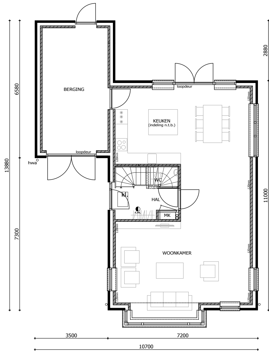
BEGANE GROND
