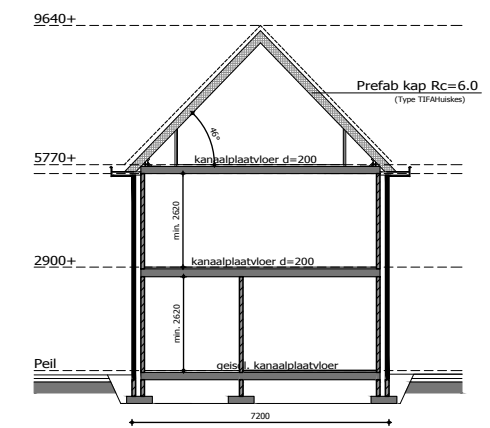
DOORSNEDE
