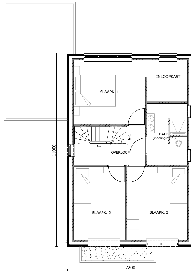
VERDIEPING
