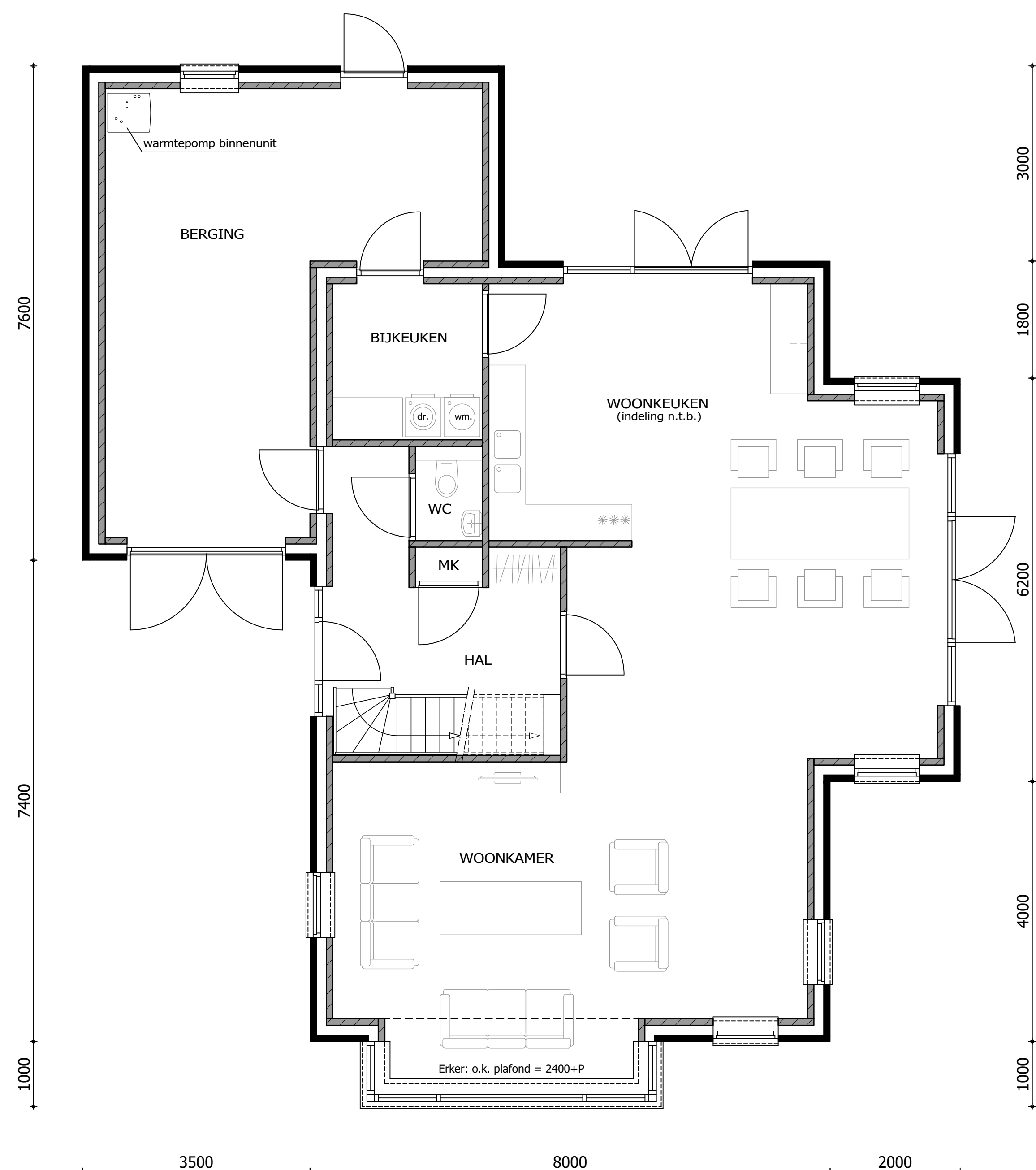
BEGANE GROND
