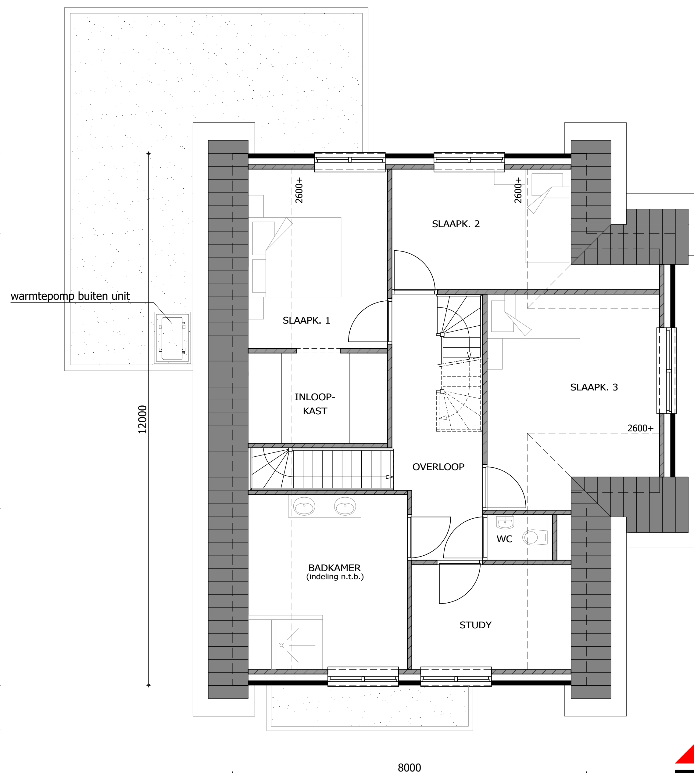
VERDIEPING
