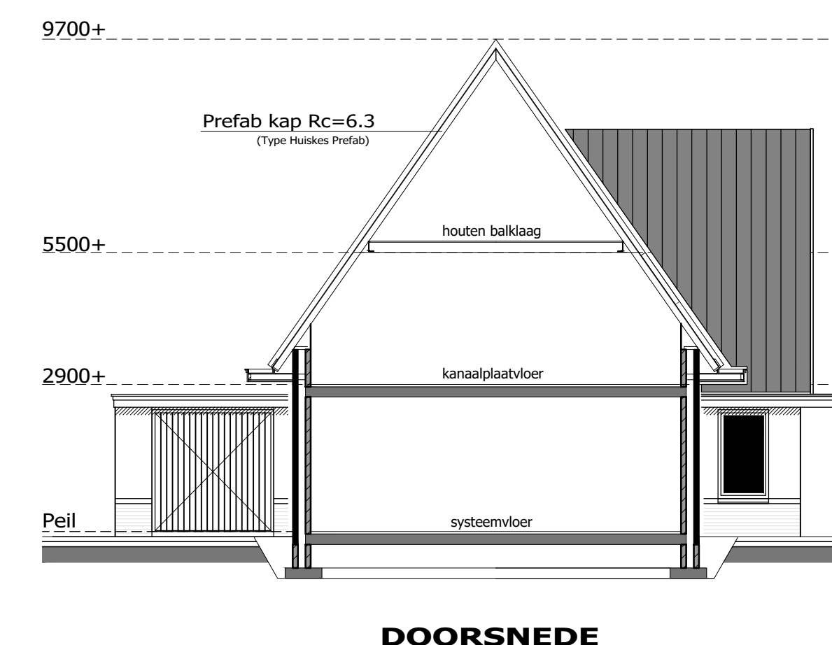
DOORSNEDE
