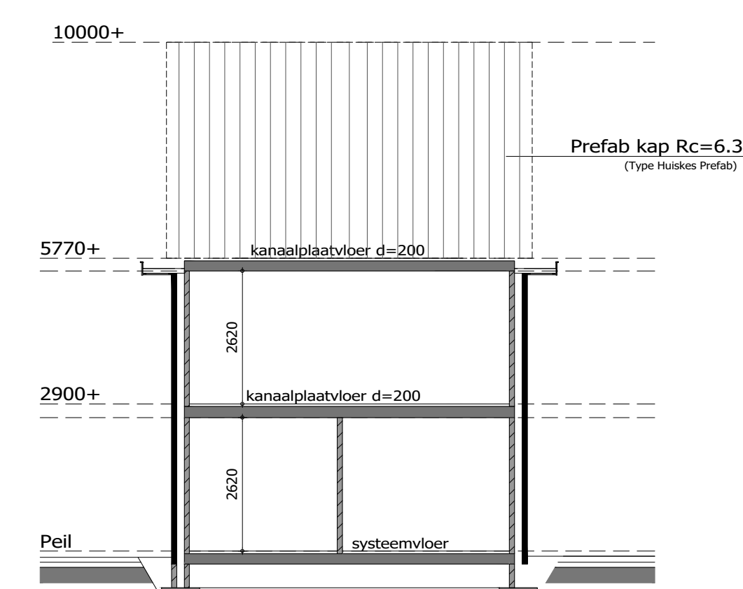
DOORSNEDE
