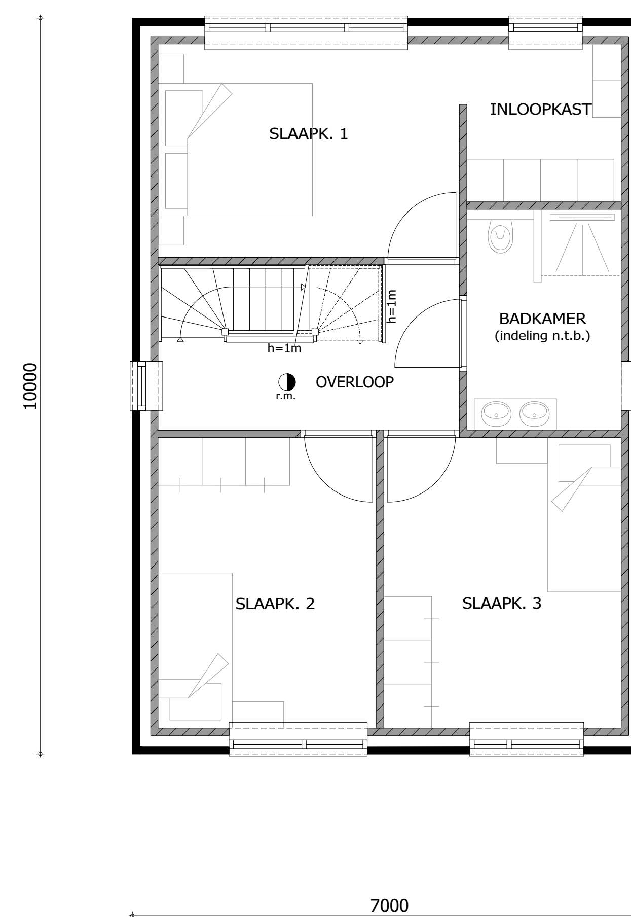
VERDIEPING
