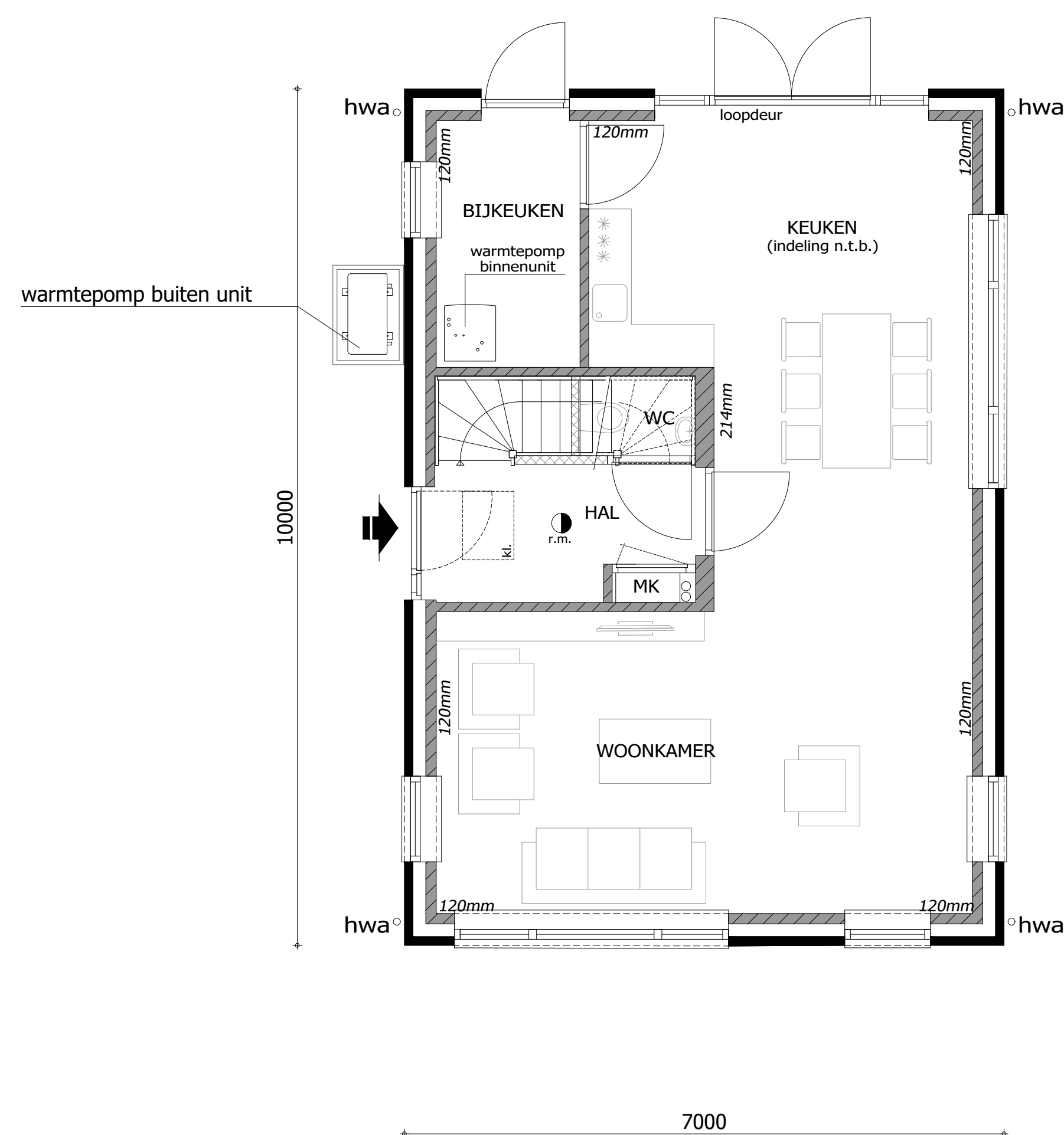
BEGANE GROND
