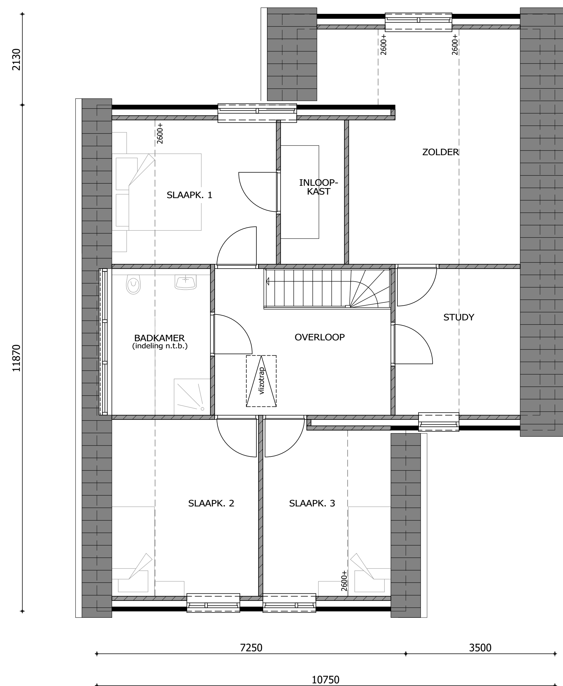
VERDIEPING
