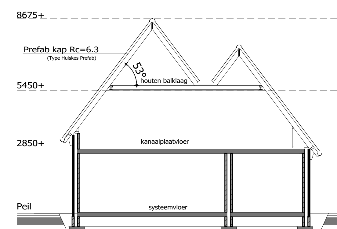
DOORSNEDE
