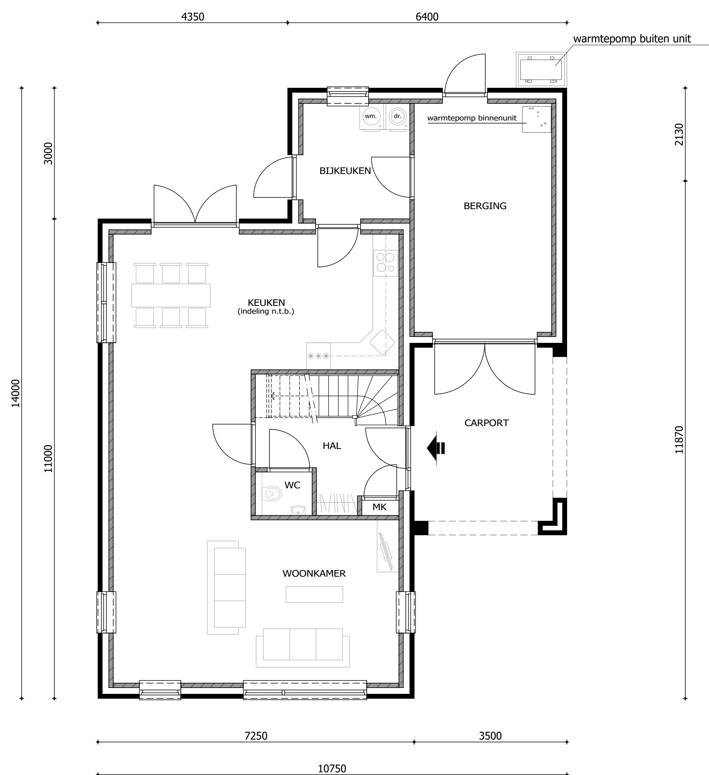
BEGANE GROND
