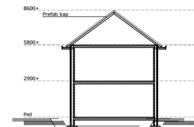
DOORSNEDE
