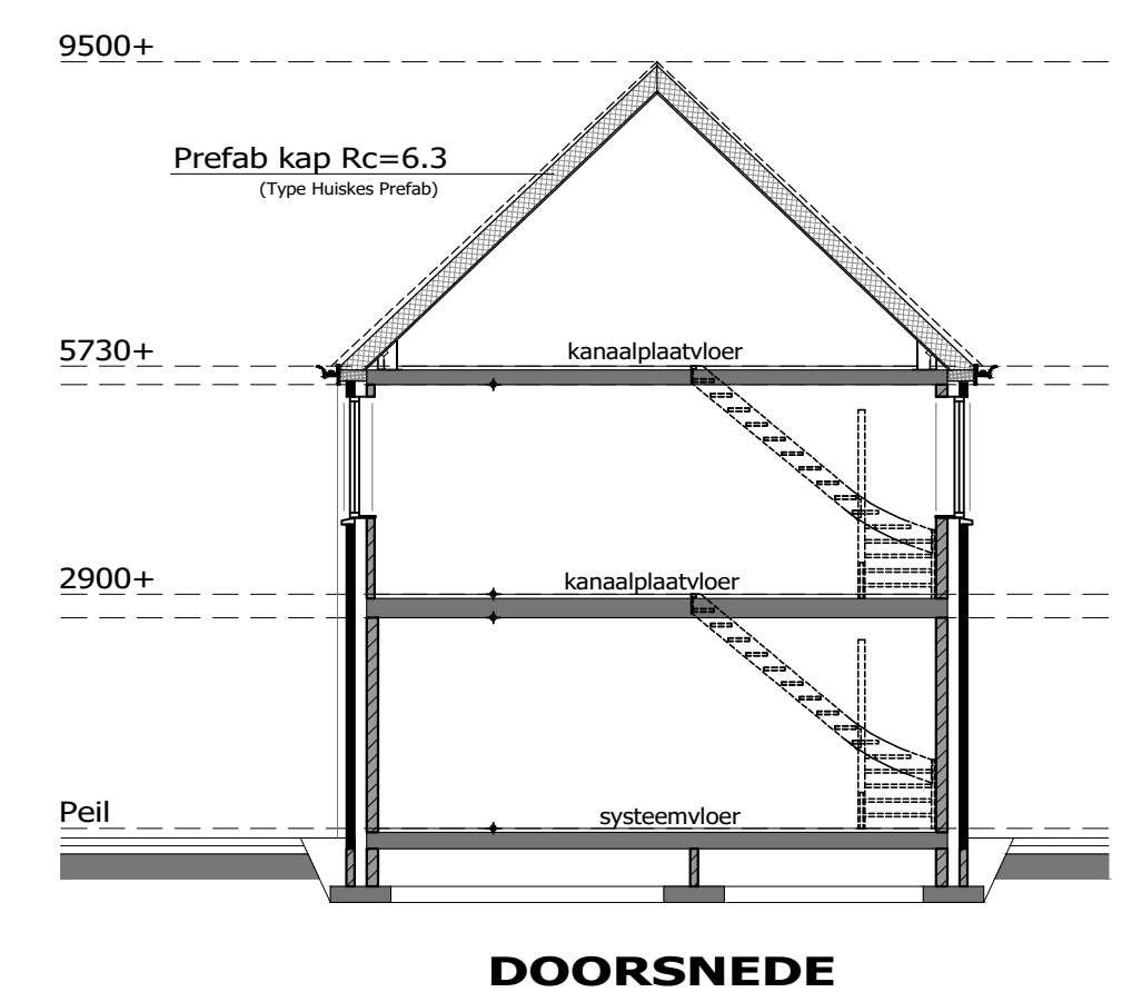
DOORSNEDE
