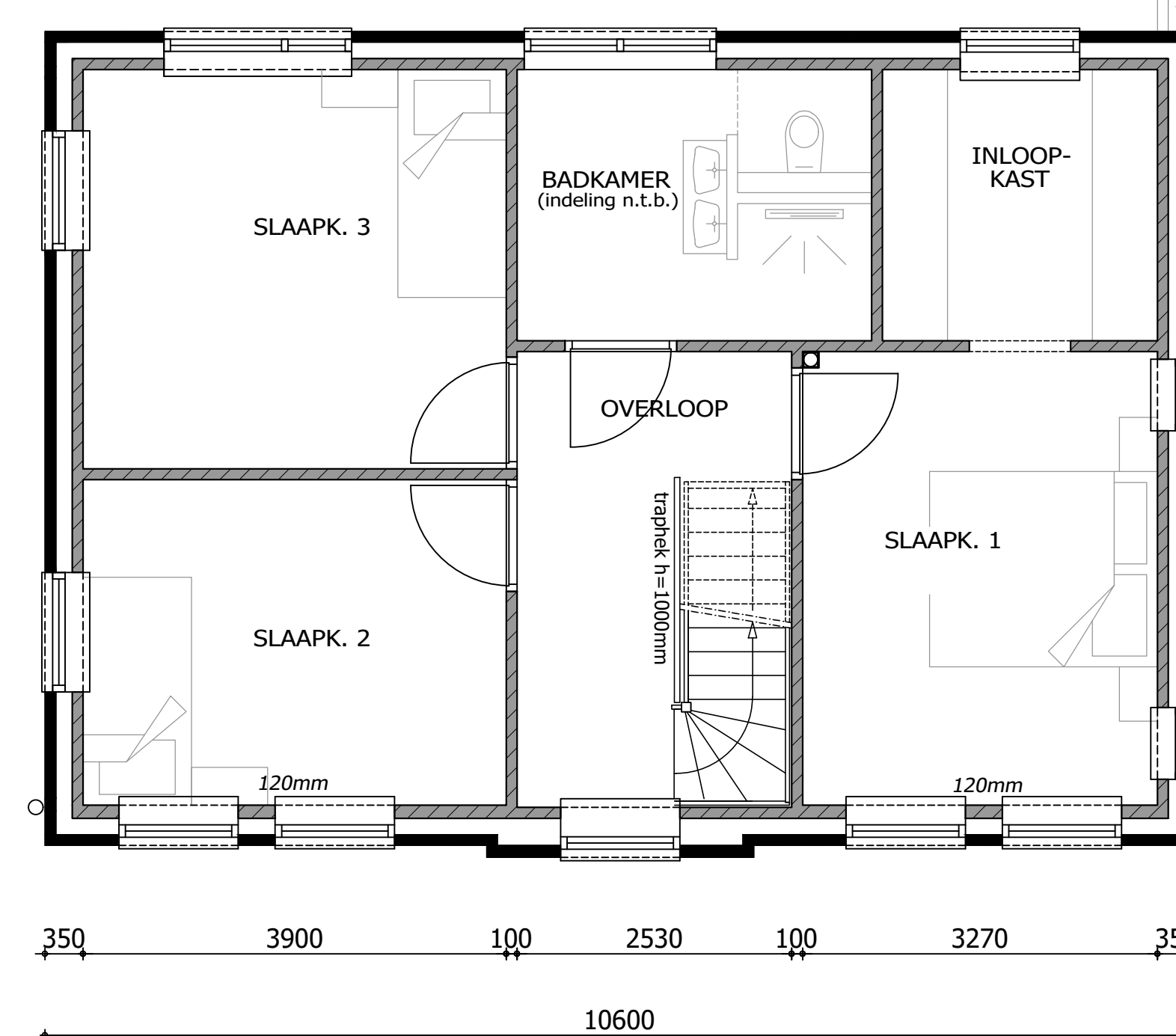
VERDIEPING
