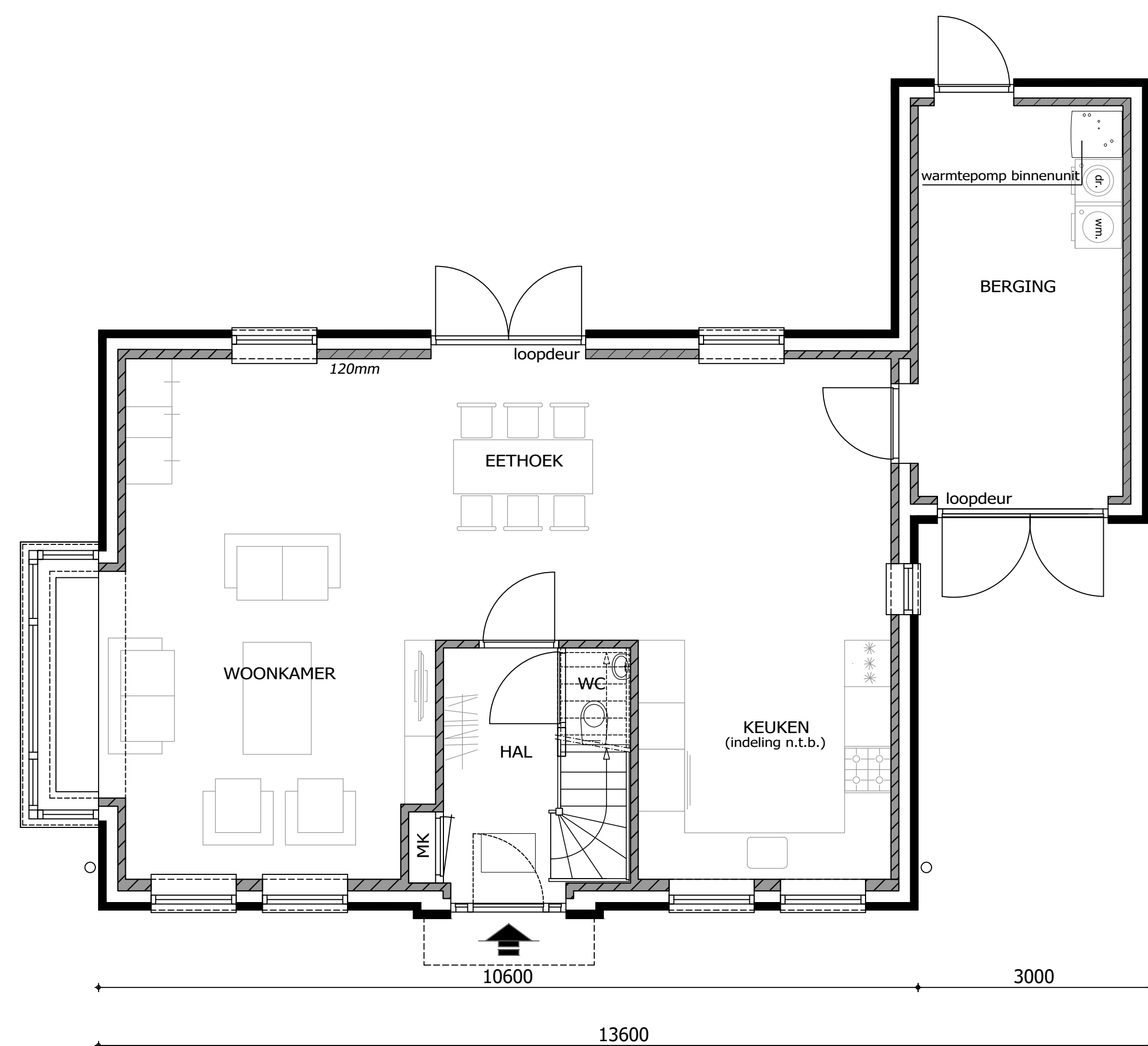
BEGANE GROND
