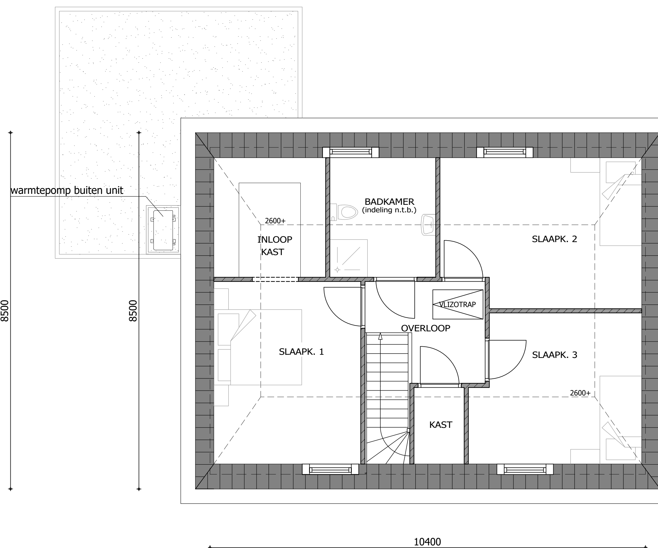
VERDIEPING
