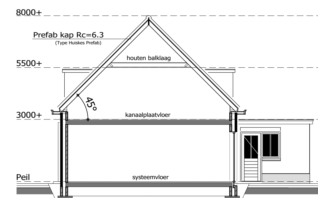
DOORSNEDE
