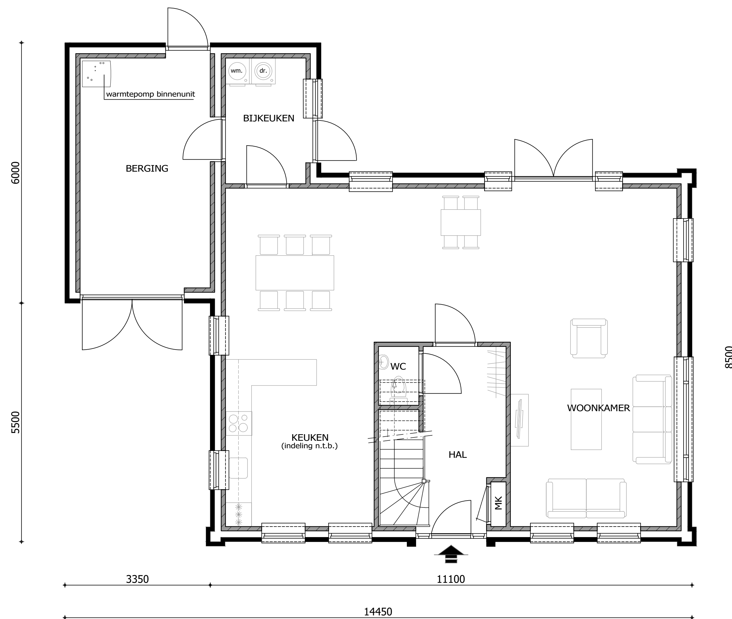
BEGANE GROND
