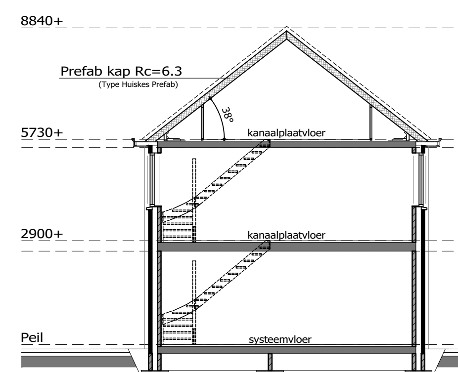
DOORSNEDE
