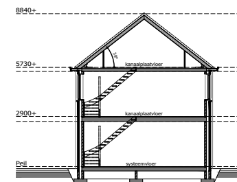
DOORSNEDE
