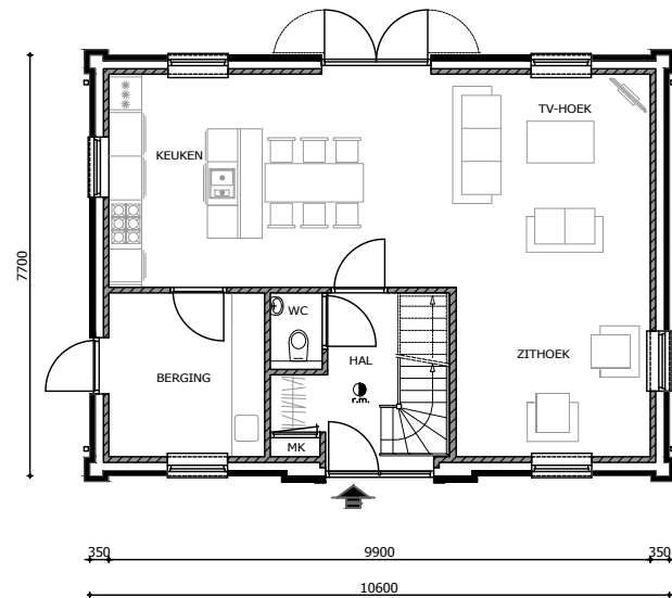
BEGANE GROND
