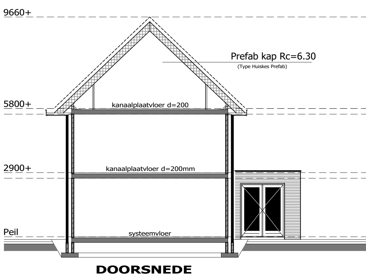
DOORSNEDE
