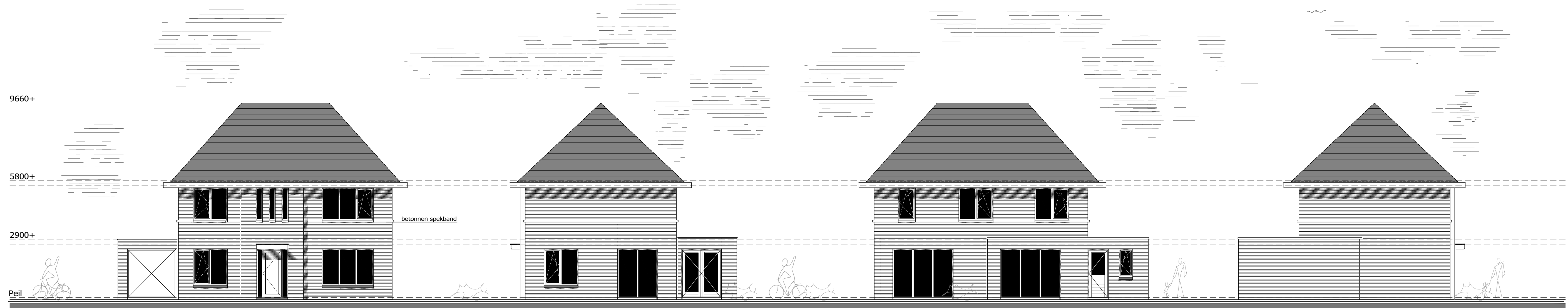
VOORGEVEL
