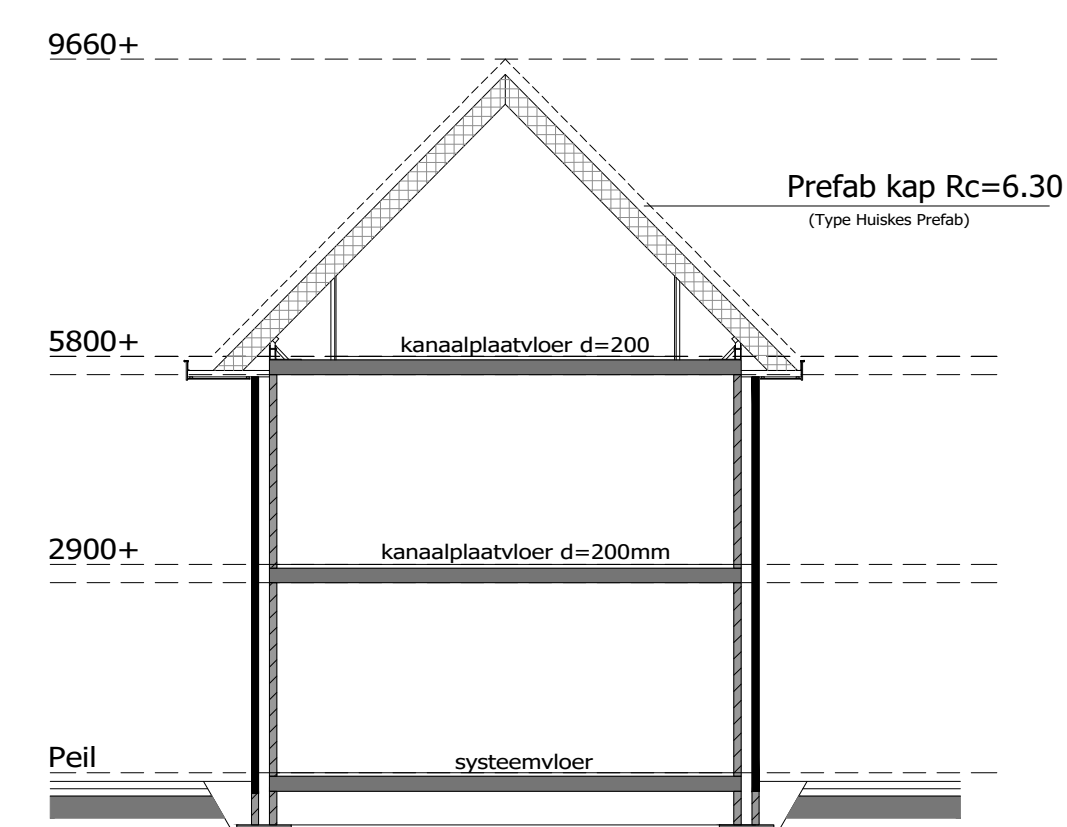
DOORSNEDE
