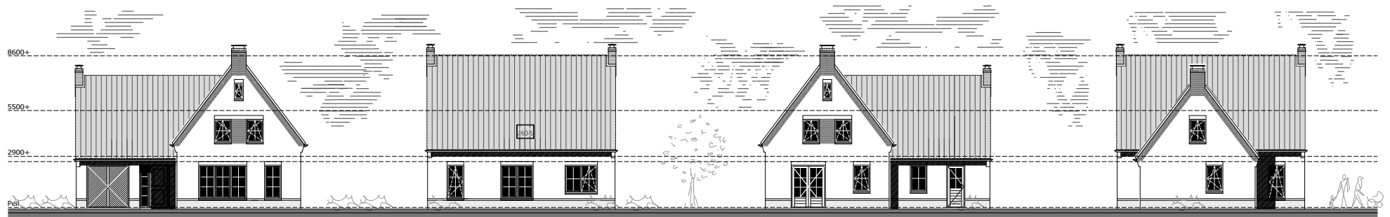
VOORGEVEL
