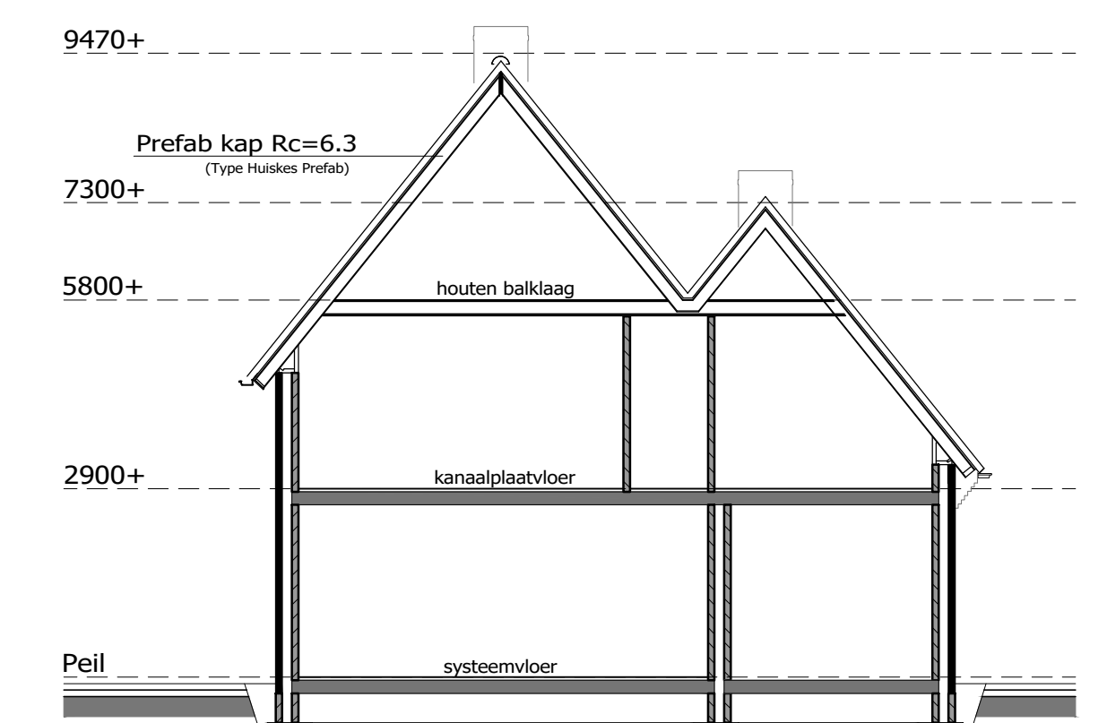
DOORSNEDE
