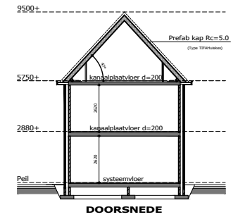
DOORSNEDE
